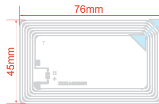
天线图 (Antenna)
